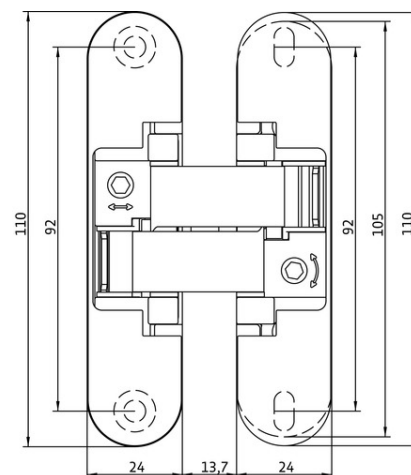
vista frontale
